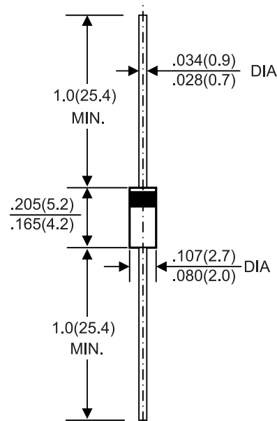
DO-204AL (DO-41)
