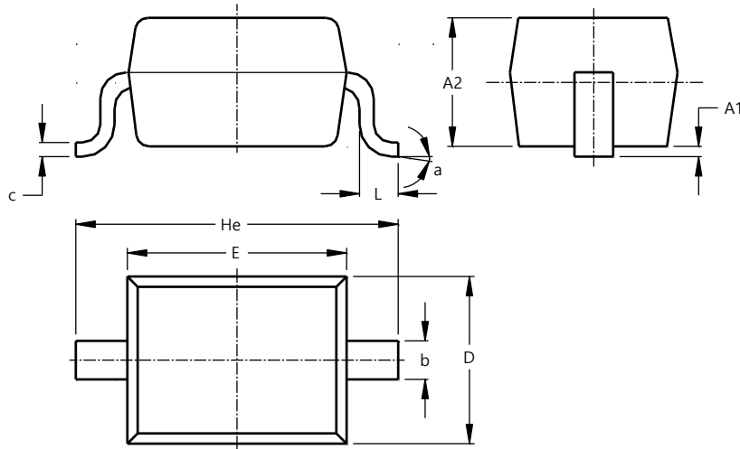
SOD323
