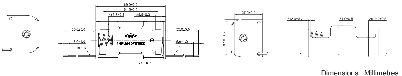
Dimensions : Millimetres
