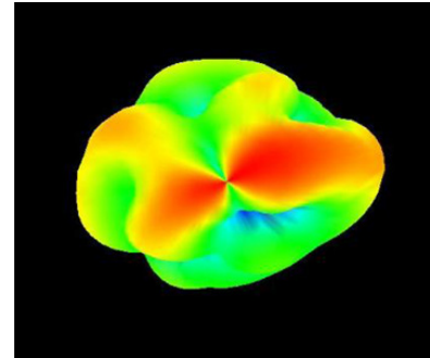
2170 MHz
