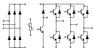
ACEPACK™ 2
