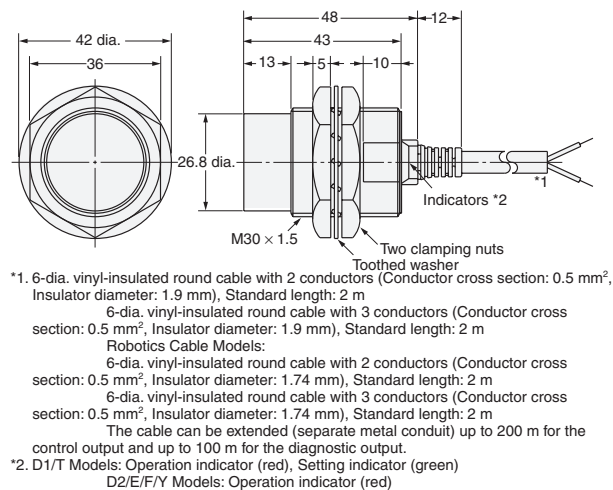
Diagram 13 E2E-X20MD□/E2E-X18ME□/F□ E2E-X18MY□
