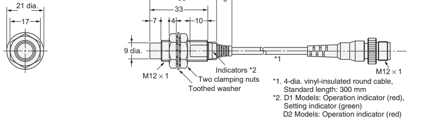
Diagram 31 E2E-X8MD1-M1GJ E2E-X8MD1-M1TGJ E2E-X8MD□-M1TGJ-US
