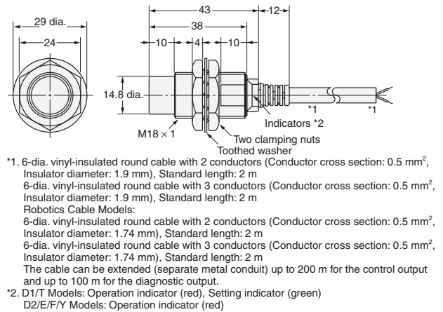
Diagram 11 E2E-X14MD□/E2E-X10ME□/F□ E2E-X10MY□
