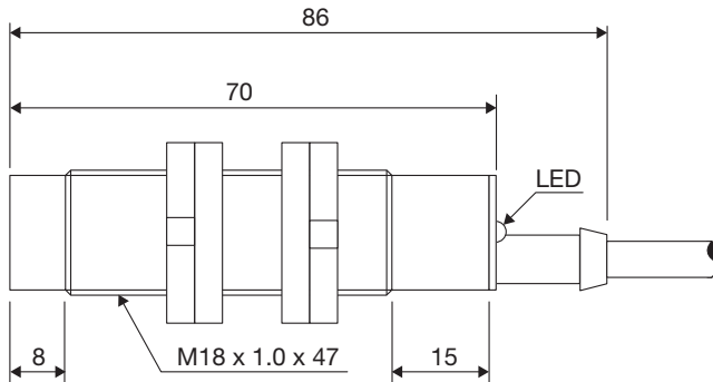
Fig. 7 Cable CA18CAN...A2IO
