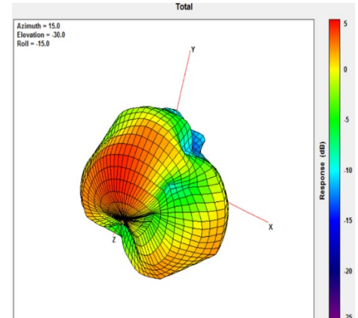
3500MHz
