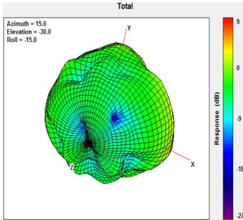
704MHz
