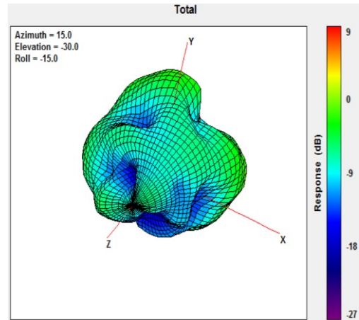
960MHz
