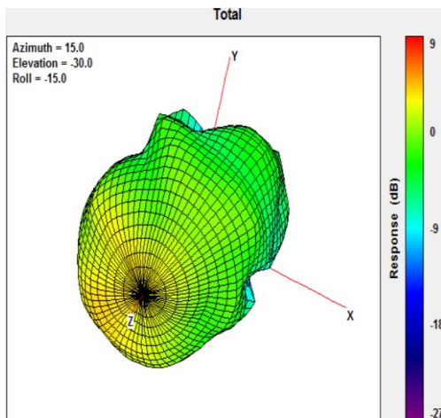
1710MHz
