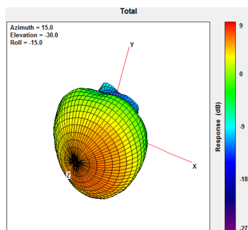
2170MHz
