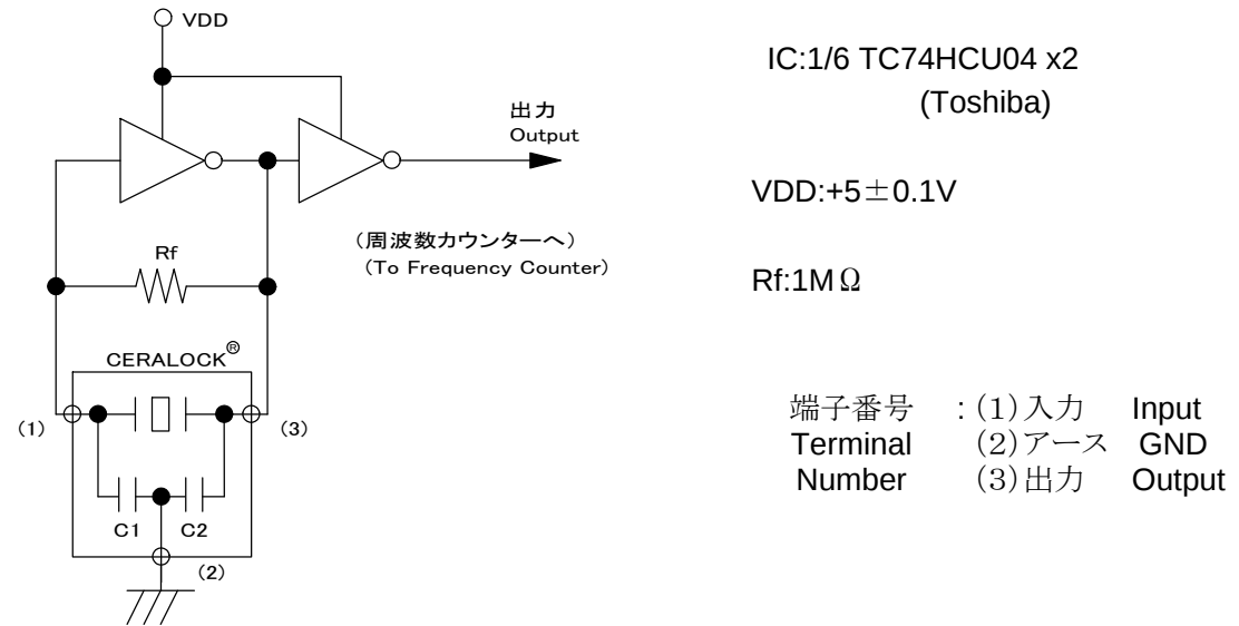
第1図 発振周波数測定回路図 Figure 1. Measurement circuit of oscillating frequency
