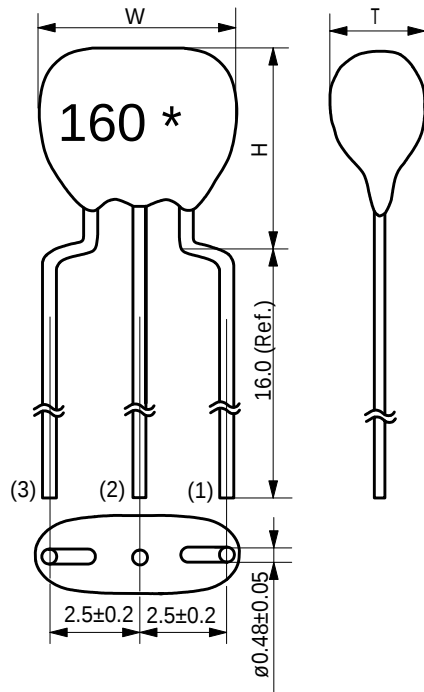
テーピング品の外形寸法図
