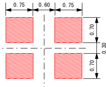
第1図 外形寸法図
