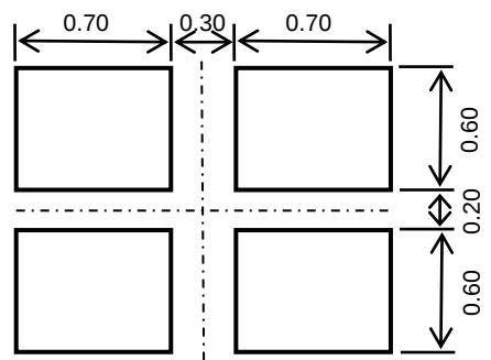
第1図 外形寸法図 Figure 1. Dimensions
