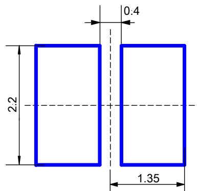
第1図 外形寸法図
