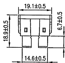
Blade Fuse Dim.
