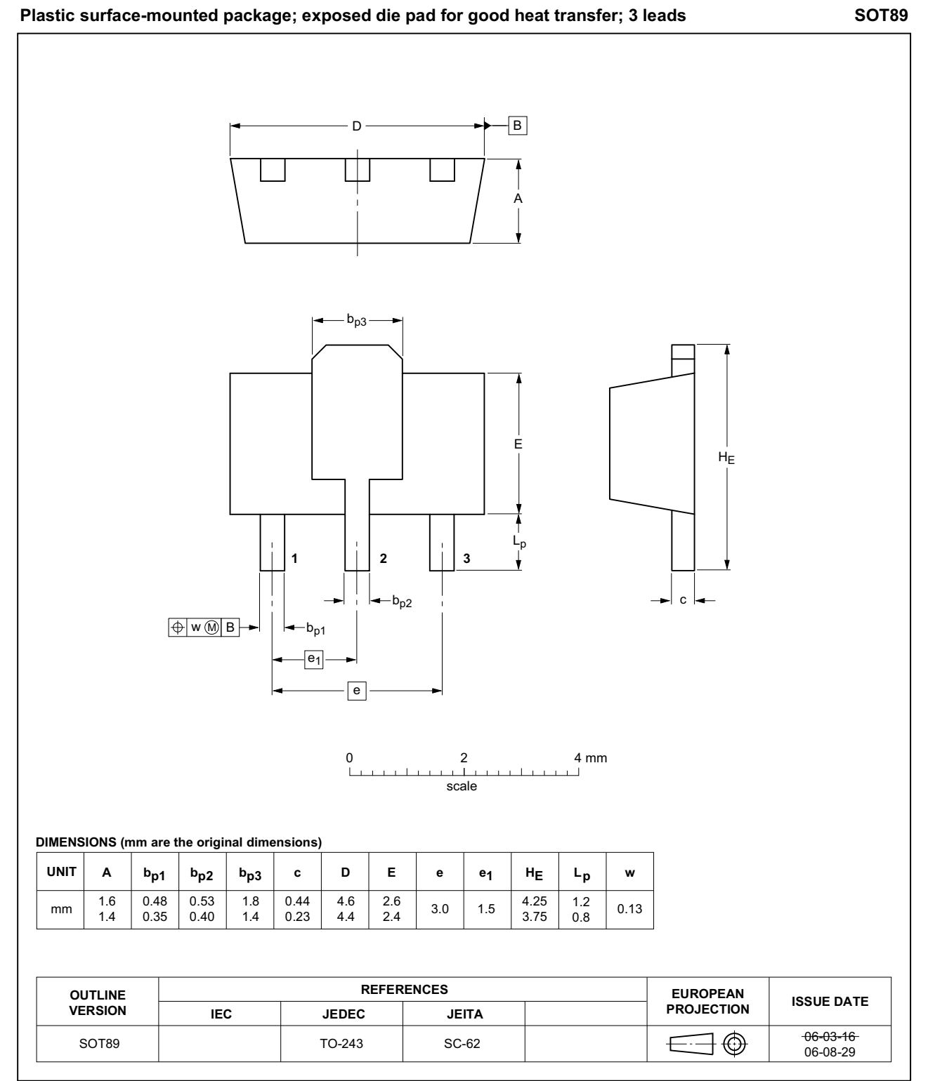
Fig 26. Package outline SOT89
