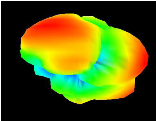
1710 MHz
