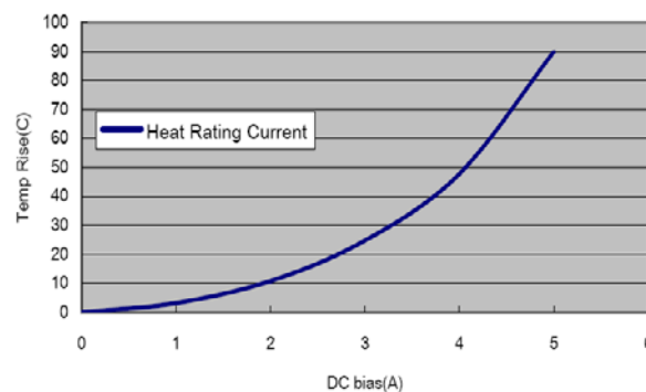
ASPI-0630LR-150
