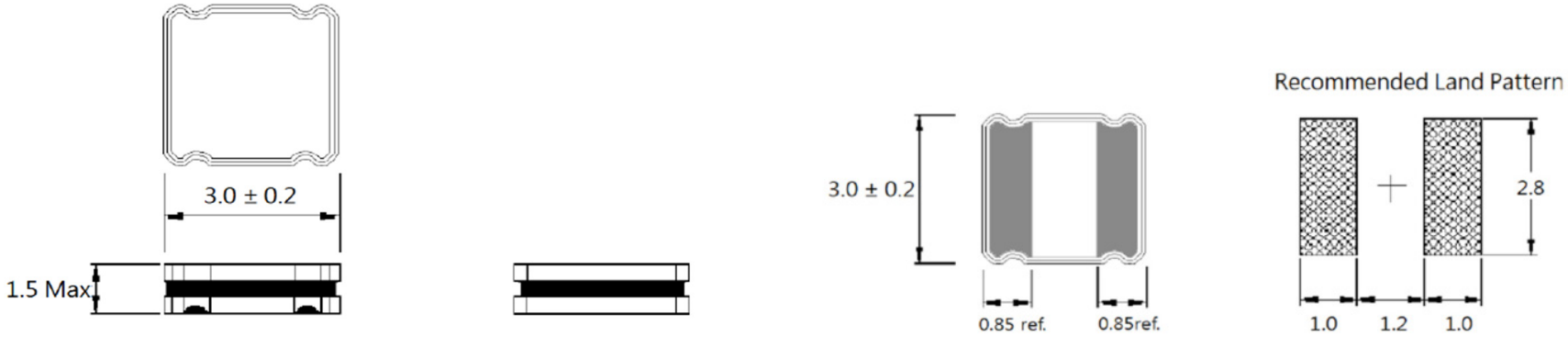
ASPI-M3015
