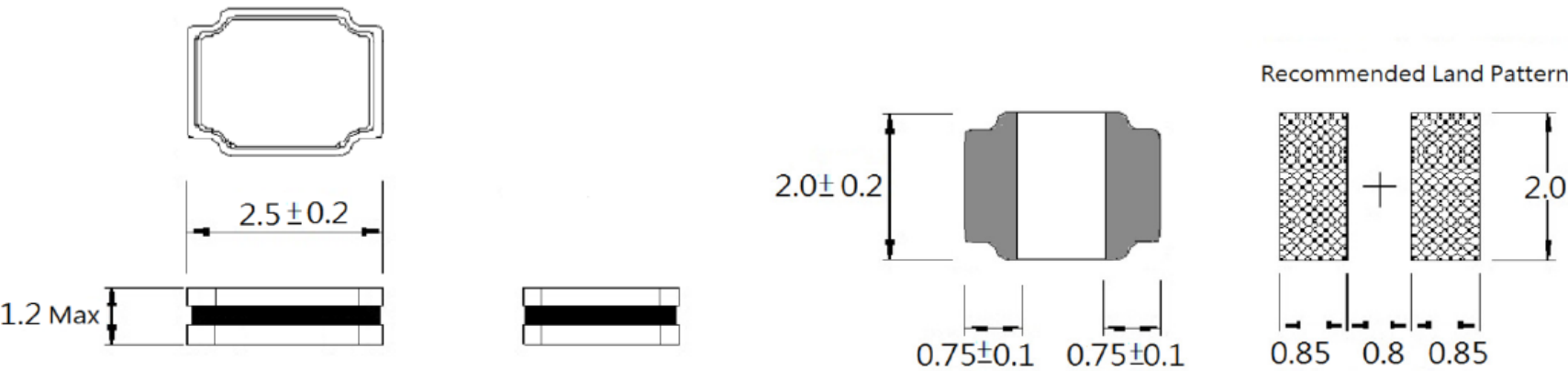
ASPI-M2512
