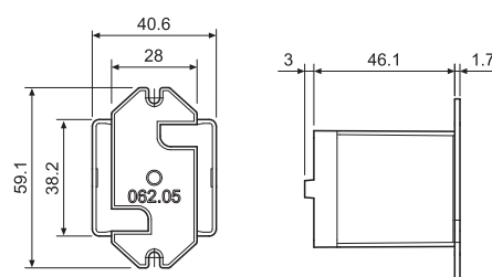
062.05
