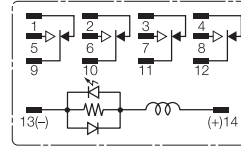
4PDT (RY4)
