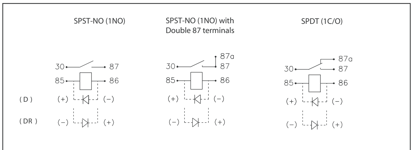
Wiring diagrams
