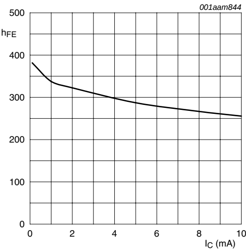
V CE = 2 V; T amb = 25 °C.
