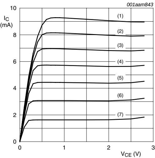
T amb = 25 °C. (1) I B = 35 μA (2) I B = 30 μA (3) I B = 25 μA (4) I B = 20 μA (5) I B = 15 μA (6) I B = 10 μA (7) I B = 5 μA
