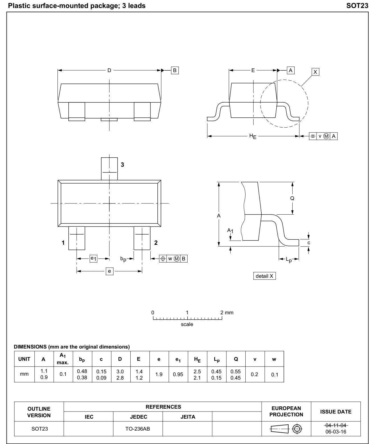
Fig 27. Package outline SOT23
