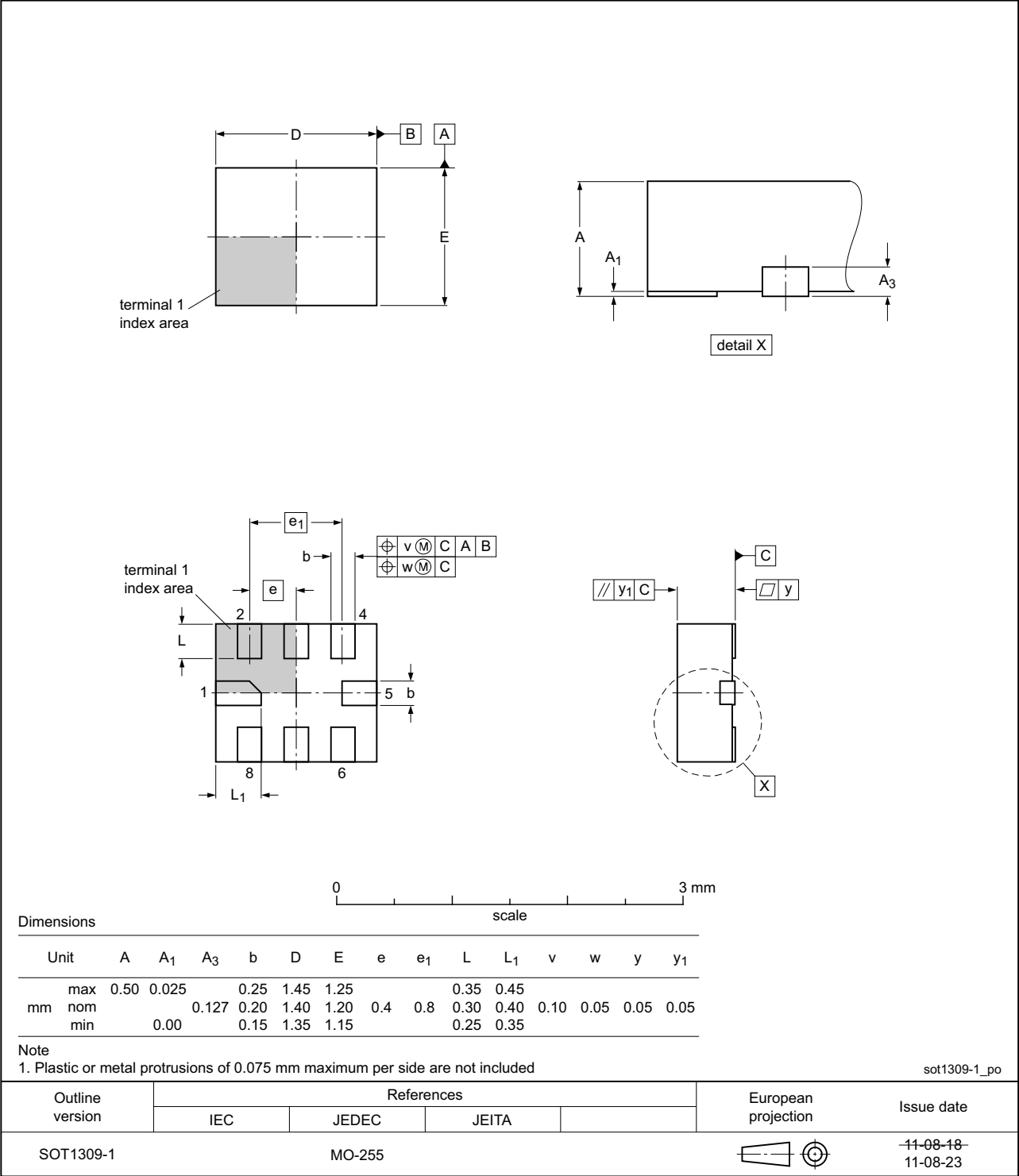
Fig 27. Package outline SOT1309-1 (XQFN8)
