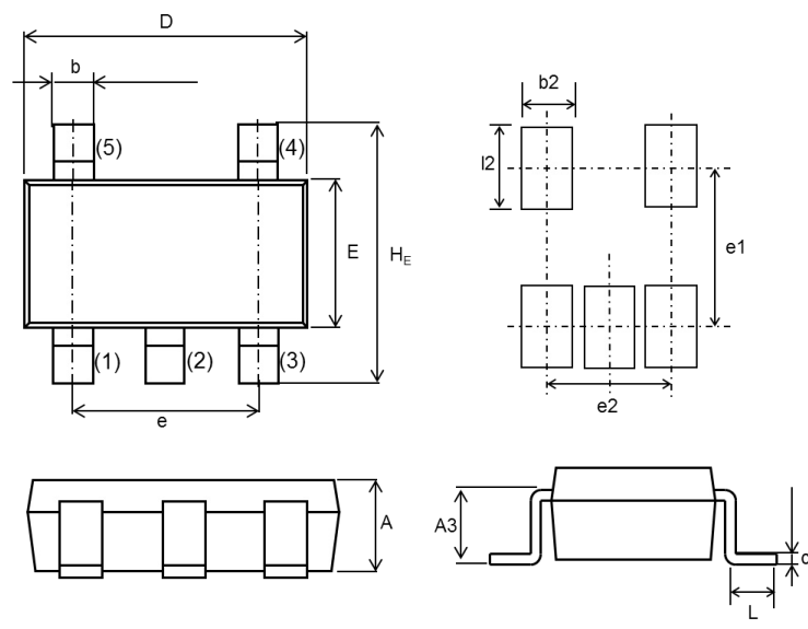
SOT-25T, (TSMD5)
