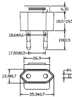
EU PIN
