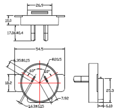
AU PIN
