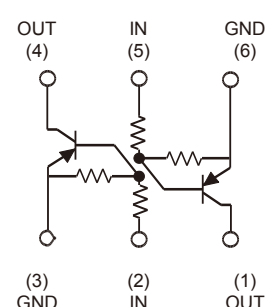
IMB10AFRA
