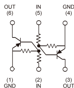
EMB10FHA / UMB10NFHA
