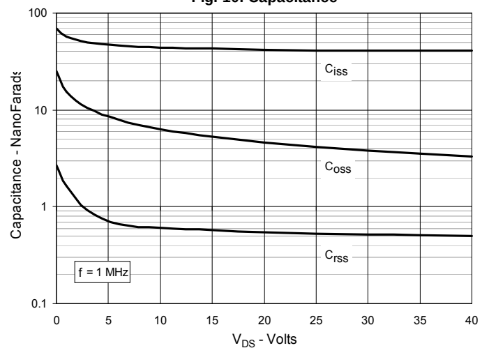
Fig. 10. Capacitance
