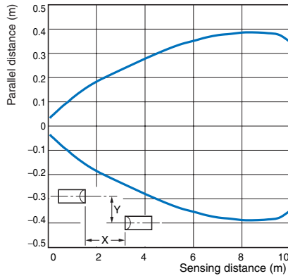
E3JK-R□□1+E39-R1S
