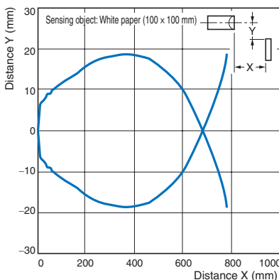
E3JK-D□□2
