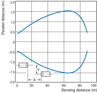
E3JK-R□□1+E39-R1
