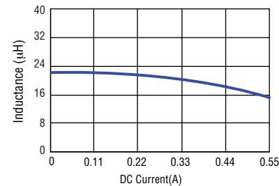
SRN3012TA-220M
