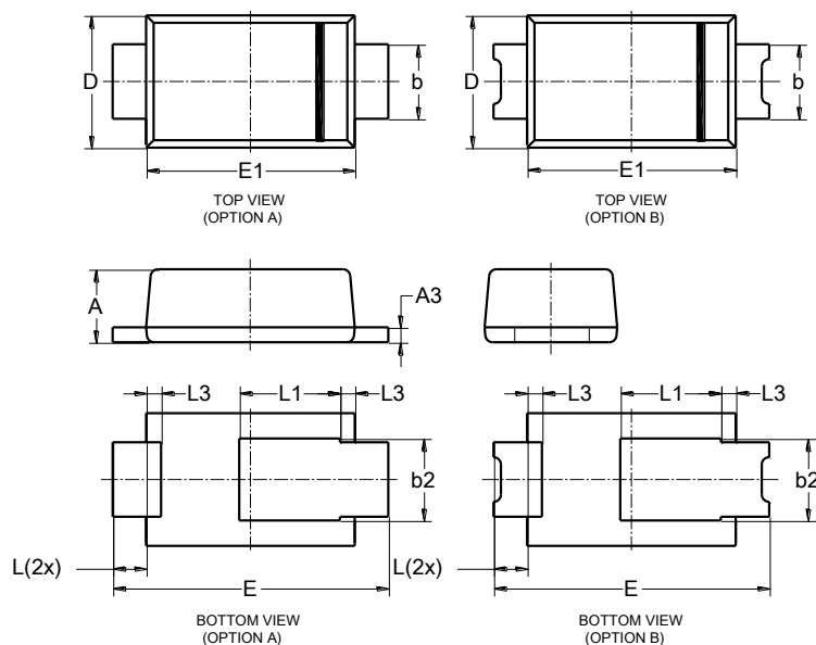
PowerDI123
