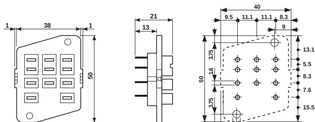
92.33
