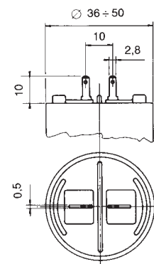
Fig. 3 Faston 2,8 x 0,5 mm
