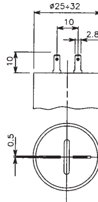
Fig. 3 Faston 2,8 x 0,5 mm
