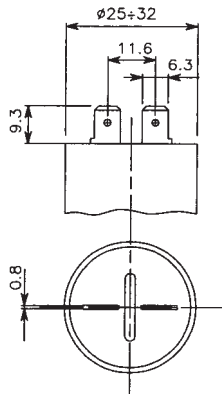
Fig. 2 Faston semplice 6,3 x 0,8 mm
