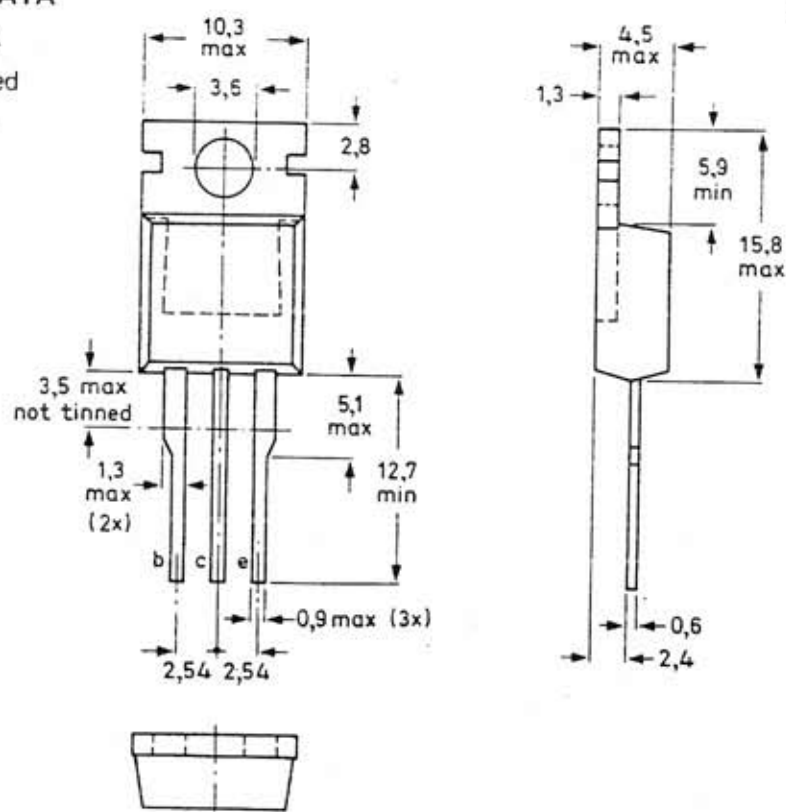
Fig. 1 TO-220AB.
