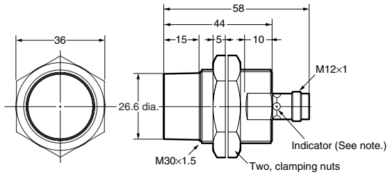
E2A-M30KN20-M1-□□/E2A-S30KN20-M1-□
