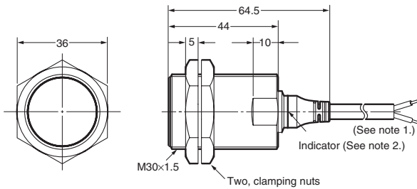
E2A-M30KS15-WP-□□/E2A-S30KS15-WP-□
