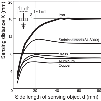
E2A-M18□N16/E2A-S18□N16
