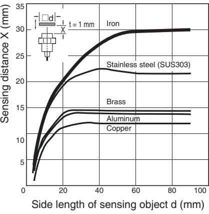
E2A-M30LN30/E2A-S30LN30
