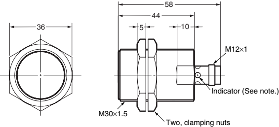
E2A-M30KS15-M1-□□/E2A-S30KS15-M1-□
