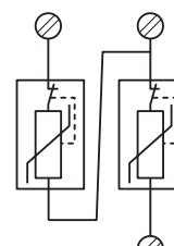
OVR 2 15 75
