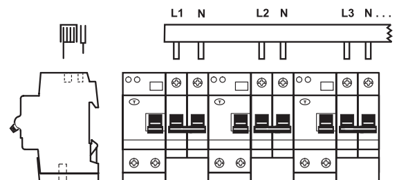
PS 4/30/16N-DDA 202 T DS 202 + DS 202 + (DDA 202 + S 202) ...
