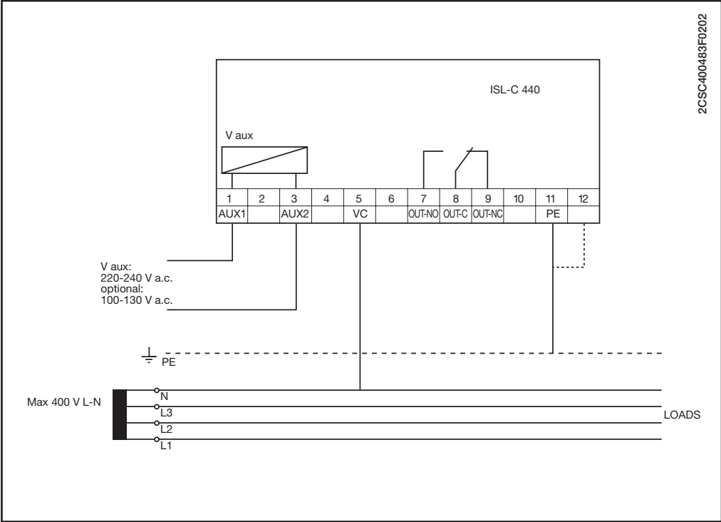
ISL-C 440
