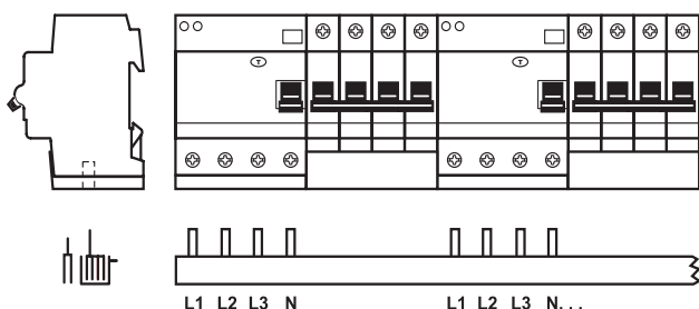
PS 3/30/16-DDA 202 T DS 202 + DS 202 + DA 202 + S 202 + DDA 202 + S 202 ...
