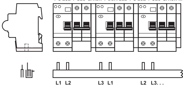
PS 4/32-DDA 204 PS 4/32/16-DDA 204 DS 204 (50/63 A) + (DDA 204 (63 A) + S 204) ...
