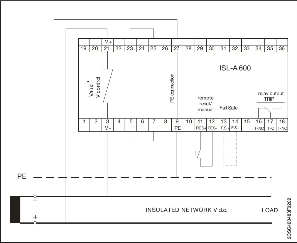
ISL-A 600
