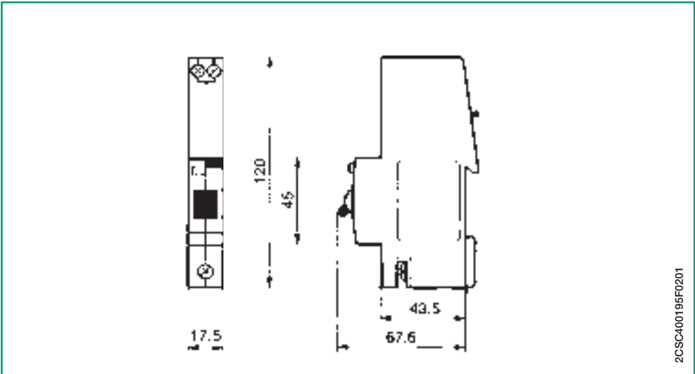
DS 271
