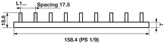
PS 1/9
