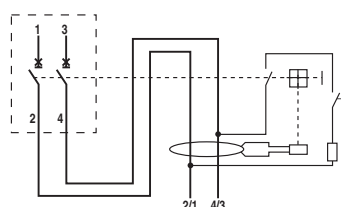
DDA 802
