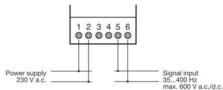
FRZ-DIG
