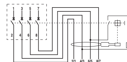
DDA 804
