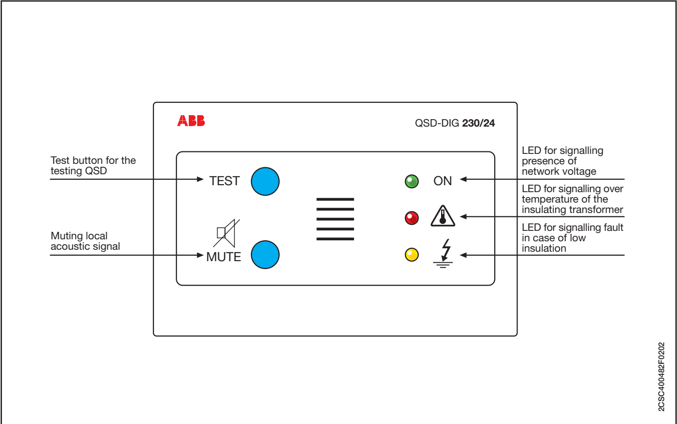
QSD-DIG 230/24
