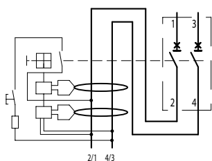
DDA 202 B type
