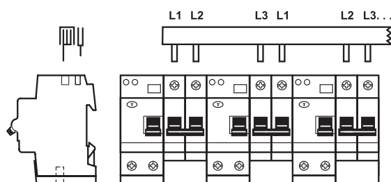
PS 3/30/16-DDA 202 T DS 202 + DS 202 + DA 202 + S 202 + DDA 202 + S 202 ...
