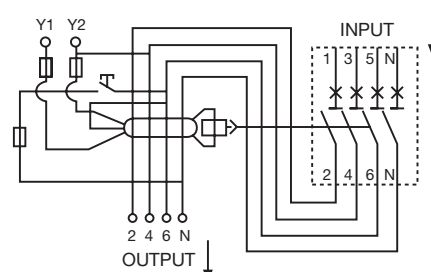
DDA 204 AE
