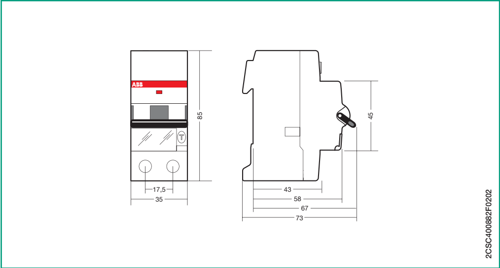
DS 271
