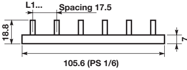
PS 1/6
