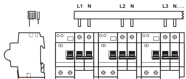
PS 4/30/16NH-DDA 202 T DS 202 + S2C-S/H6R + DS 202 + S2C-S/H6R + (DDA 202 + S 202) + S2C-S/H6R + (DDA 202 + S 202) + S2C-S/H6R ...
