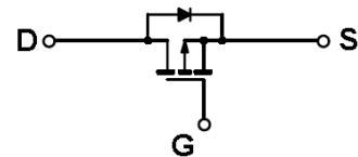
P-Channel MOSFET
