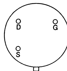
TO18
