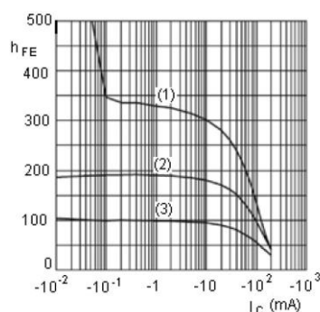
BC857A : V_{CE} = -5V
