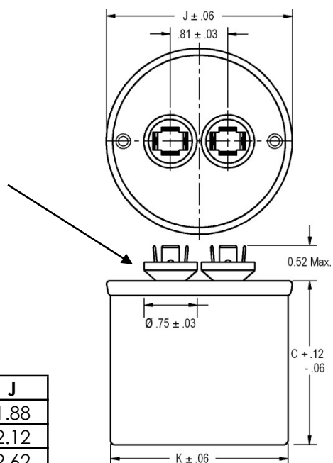
Case Style P, S, and T
