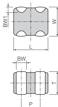
[2 Array Type]
