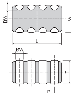
[4 Array Type]
