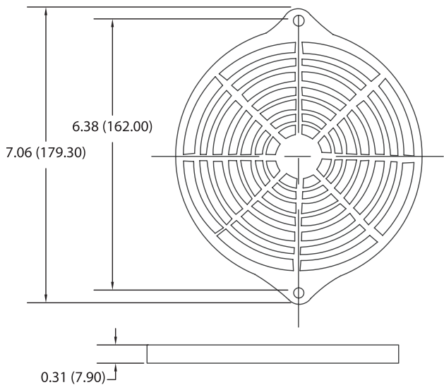
Dimensions : Inches (Millimetres)
