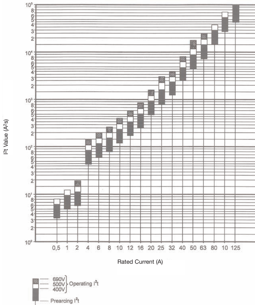
Class gG/gL - I^2t Values
