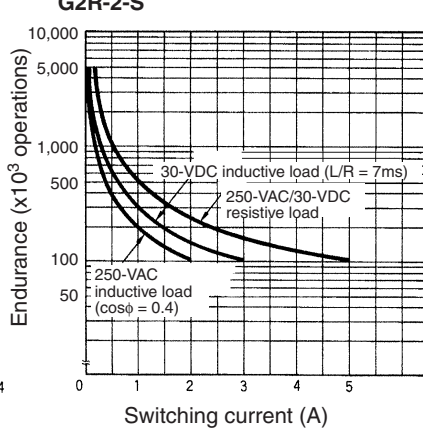
G2R-2-S
