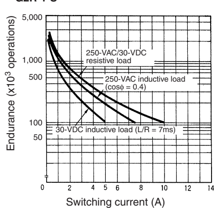
G2R-1-S
