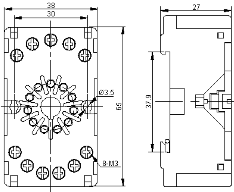
Dimensions : Millimetres
