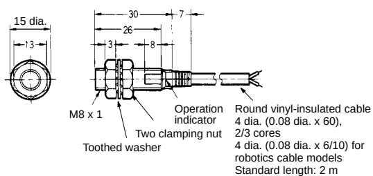
Fig. 6 : E2E-X1R5Y□
