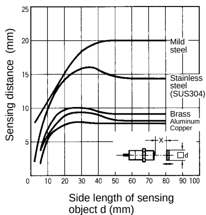
E2E2-X20MD□
