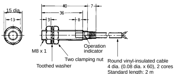
Fig. 8 : E2E-X3D□-N E2E-X2E□/F□
