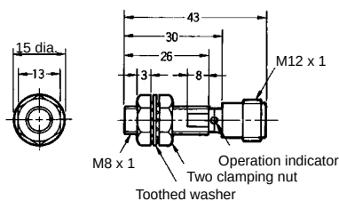
Fig. 17 : E2E-X2D□-M1G E2E-X1R5E□-M1/F□-M1
