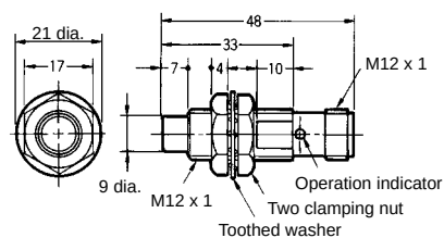
Fig. 20 : E2E-X8MD□-M1G E2E-X5ME□-M1/F□-M1
