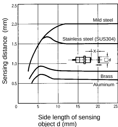
E2E2-X5C□/B□ E2E2-X5Y□
