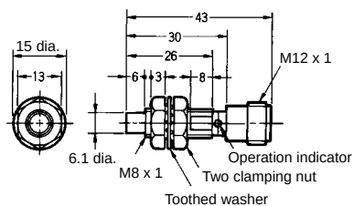
Fig. 18 : E2E-X4MD□-M1G E2E-X2ME□-M1/F□-M1
