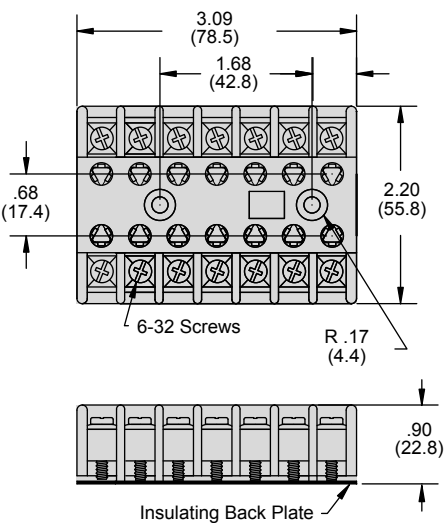
14 Pin Socket - 33377
