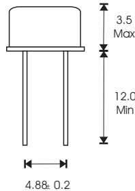
HC-49/S
