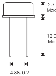
HC-49/SS
