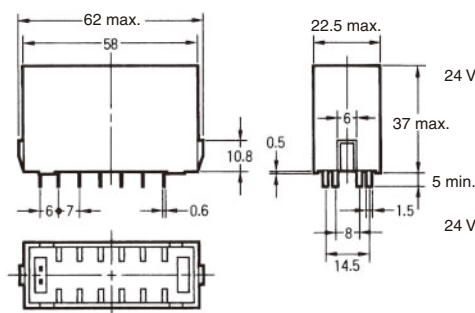
G7S-3A3B
