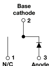
TO-263AB (D²PAK)
